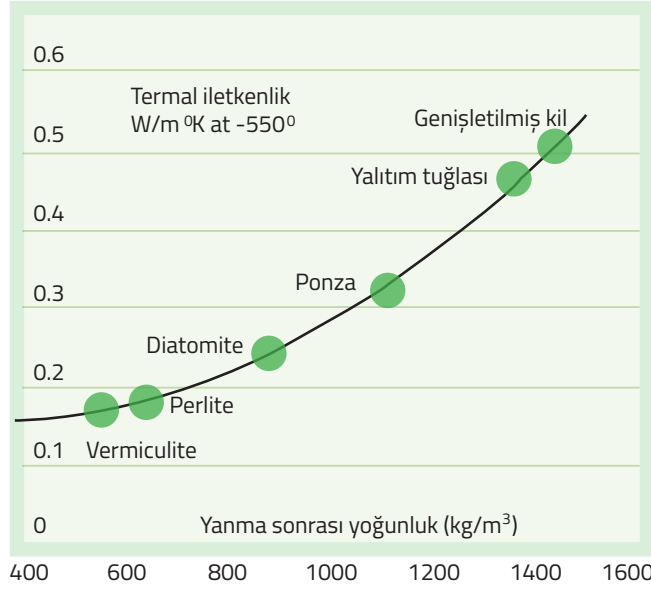
Şekil 3: Isı dirençli yalıtım betonlarının ısı iletkenlik-yakma sonrası yoğunluk ilişkisi.
