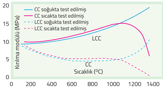
Şekil 5. Geleneksel ve LCC betonuna ait kırılma modülü
