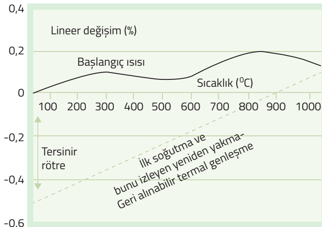
Şekil 4: Betonun ısıtma ve soğutma çevrimi
